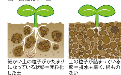
図 団粒化した土
